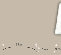
CT-2478 YATAY BANT ARMATÜR
