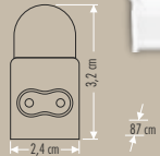
CT-2469 T5 BANT ARMATÜR BEYAZ KASA EKLENEİLİR ANAHTARLI
